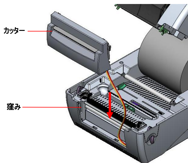
図 26 カッターモジュールの取り付け
