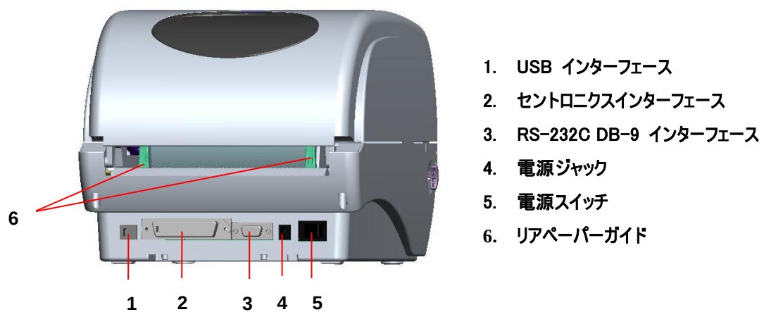
図2 背面
