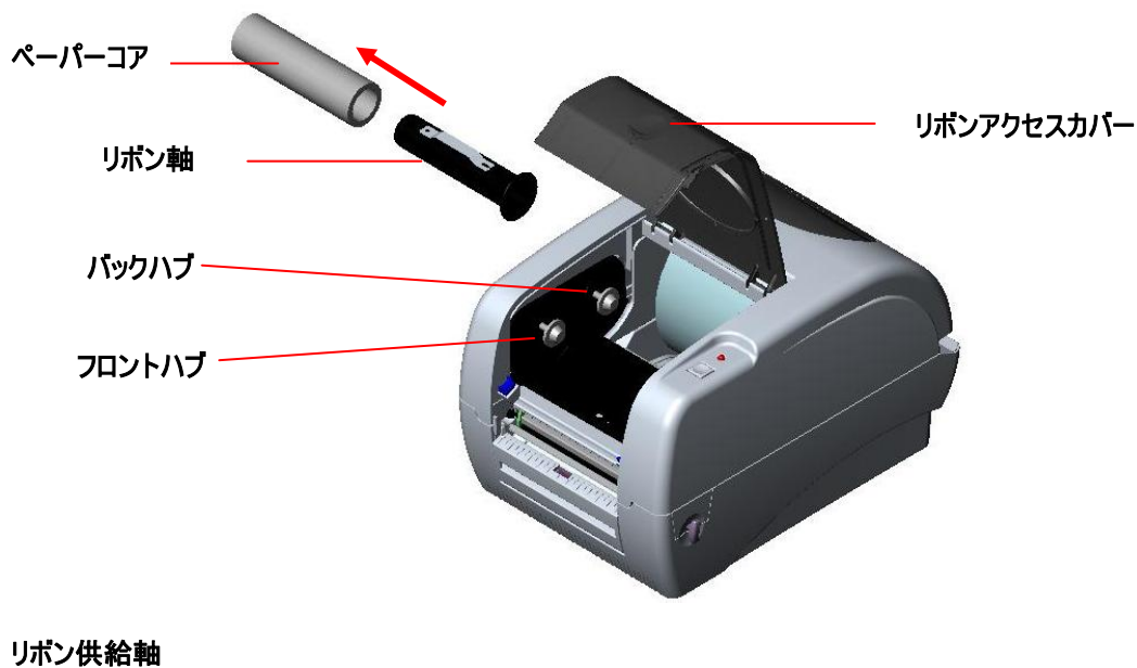
図 4 リボンの取り付け (I)
