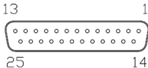
Dsub25 ピン 接続
